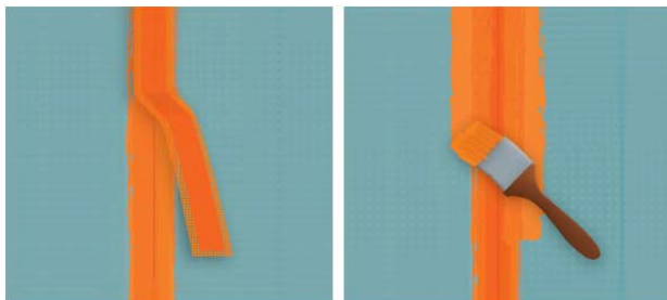
Application de la bande de pontage dans la première couche de SPEC encore fraîche et passe de la seconde couche de SPEC sur la bande mise en place.
